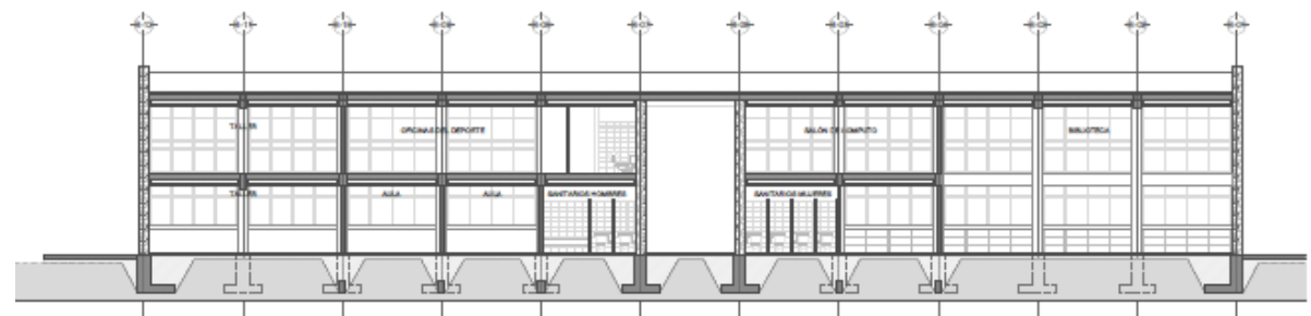
Corte Longitudinal
