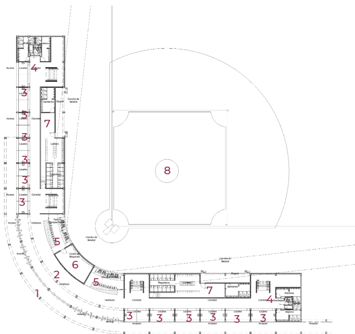
Planta Baja Edif. A
