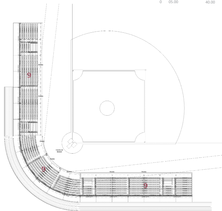
Planta Alta Edif. A
