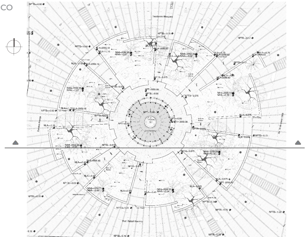
Planta Baja
