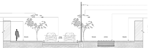
Sección de calles
