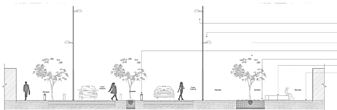
Sección de calles principales
