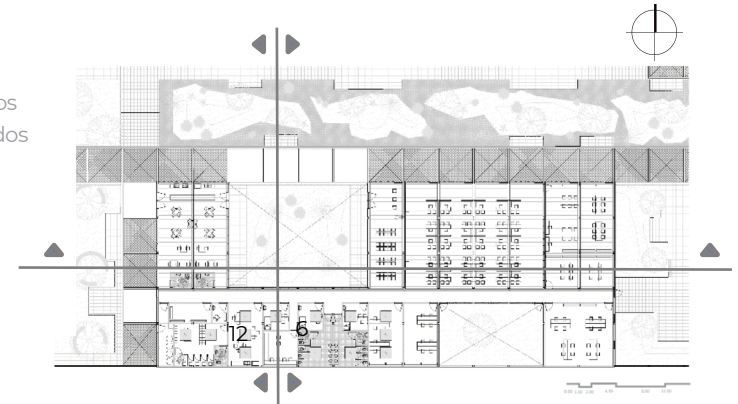
Planta Baja | Centro de Desarrollo Social
